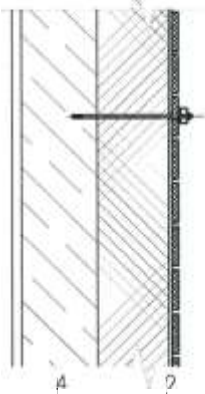
Схема узла крепления конструкции
